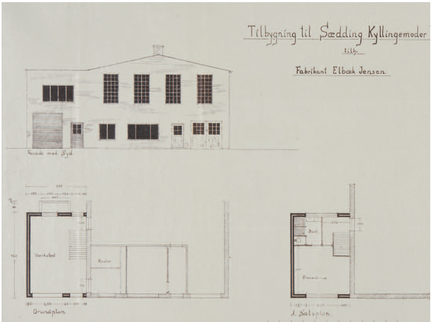
Tegning til tilbygning til Esbjerg Kyllingemoderfabrik fra oktober 1948. EBA 110297-109
